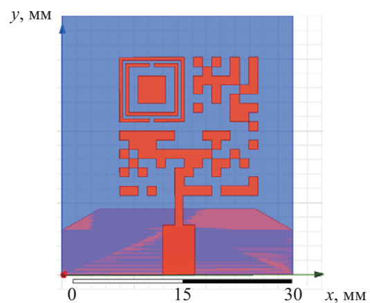
Рис. 2. Конструкція патч-антени.
